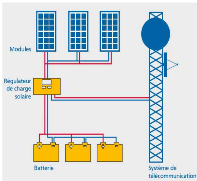
Schéma du fonctionnement d'une station énergie autonome reliée à un système télécoms
