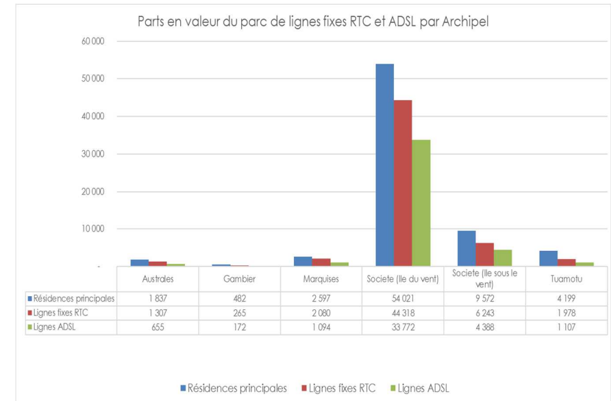
Taux de couverture OPT en fixe par archipel (EN VALEUR)
