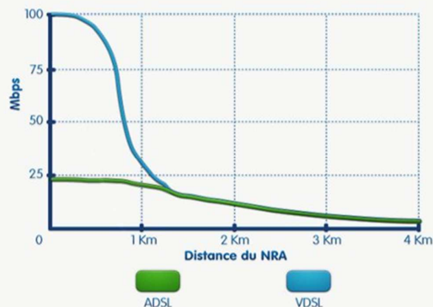
Download théorique en fonction de la distance NRA/modem
